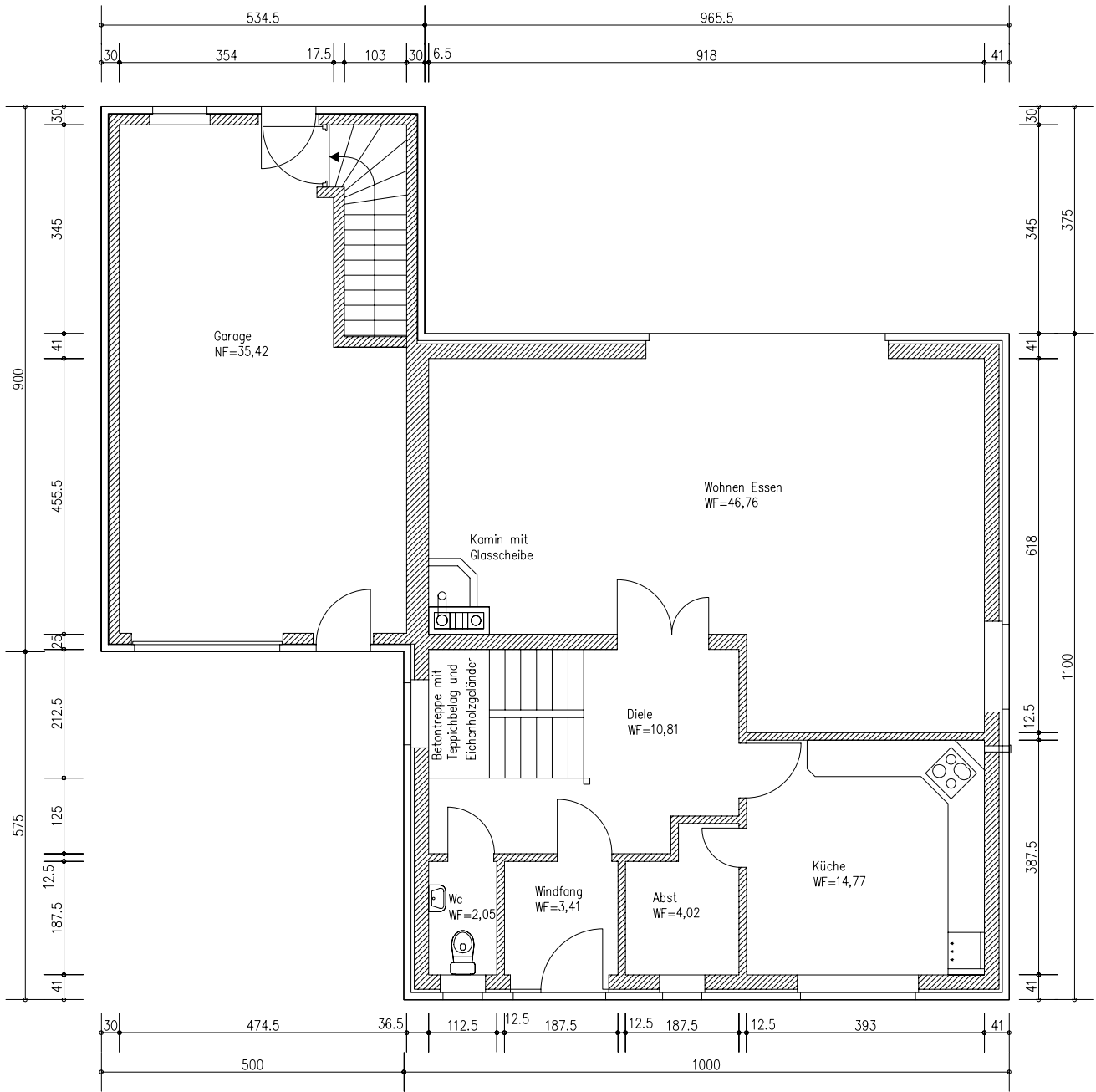
Erdgeschoß
